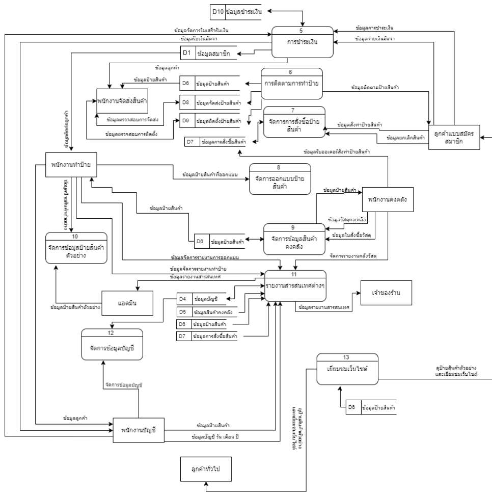
ภาพที่ 3.5 แผนภาพกระแสข้อมูลระดับที่ 0 (Data Flow Diagram Level 0)
