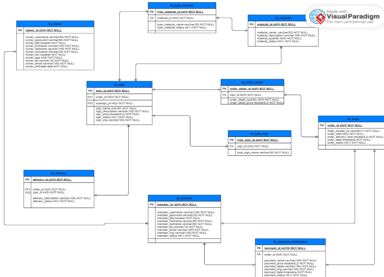
ภาพที่ 3.6 แสดงแผนผังความสัมพันธ์ข้อมูล (E-R Diagram)
